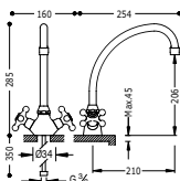
Bimando fregadero vertical CLASIC caño de tubo de 210 mm.
