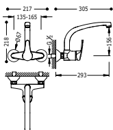
Monomando fregadero pared ECO
