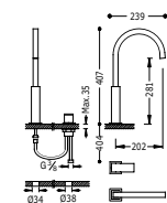
Monomando de repisa CUADRO caño de 22x22 mm.
