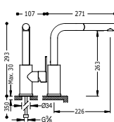
Monomando fregadero vertical LEX con ducha extraíble
