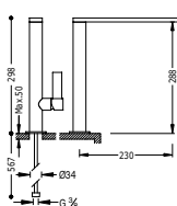
Monomando fregadero vertical CLASS caño de 34x9 mm.
