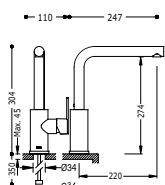
Monomando fregadero vertical LEX
