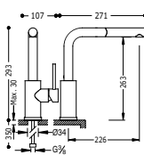
Monomando fregadero vertical MAX con ducha extraíble
