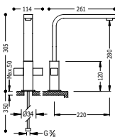
Bimando fregadero vertical CUADRO caño de 35x15 mm.
