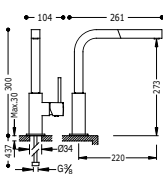
Monomando fregadero vertical CUADRO con ducha extraíble.
