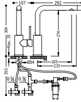
Monomando fregadero vertical doble función con filtro
