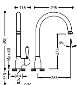
Monomando fregadera vertical RETRO con rociador extraíble
