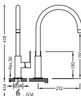
Monomando fregadero vertical LOFT
