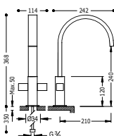
Bimando fregadero vertical CUADRO caño 35x15 mm, con aireador rectangular oculto
