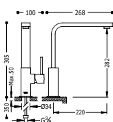
Monomando fregadero vertical CUADRO caño de 35x15 mm.
