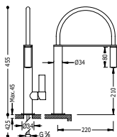
Monomando fregadero vertical CLASS con rociador extraíble.
