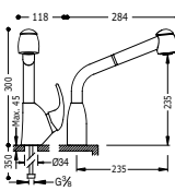
Monomando fregadero vertical con ducha extraíble (2 funciones)
