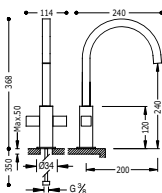
Bimando fregadero vertical CUADRO caño de 22x22 mm.
