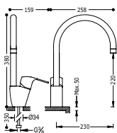
Monomando fregadero vertical K
