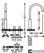
Bimando de repisa CUADRO caño de 22x22 mm.
