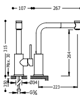
Monomando fregadero vertical MAX con ducha extraíble (2 funciones)
