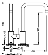
Monomando fregadero vertical MAX
