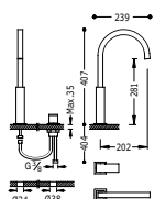
Monomando de repisa CUADRO caño de 22x22 mm.
