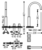
Bimando de repisa CUADRO caño de 22x22 mm.
