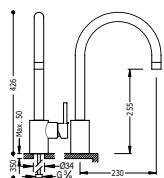
Monomando fregadero vertical MAX
