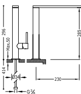
Monomando fregadero vertical MAX caño de 34x9 mm.
