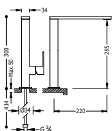
Monomando fregadero vertical CUADRO caño de 34x10 mm.
