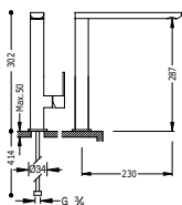
Monomando fregadero vertical LOFT caño de 34x15 mm.
