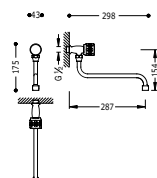
Grifo fregadero giratorio de 1/2" ESE-23
