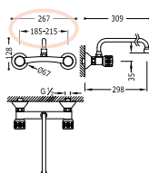
Grupo fregadero pared ESE-23
