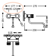
Grupo fregadero pared ESE-23 Distancia a pared de 258 mm.
