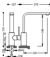
Monomando fregadero vertical caño de 35x15 mm
