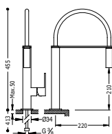
Monomando fregadero vertical CUADRO con rociador extraíble.
