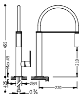
Monomando fregadero vertical MAX con rociador extraíble
