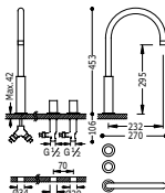
Bimando de repisa STUDY
