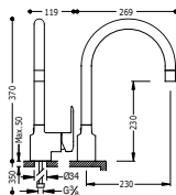
Monomando fregadero vertical con rociador extraíble
