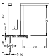
Monomando fregadero vertical LOFT caño de 34x15 mm.
