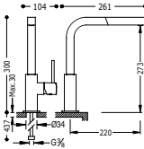
Monomando fregadero vertical CUADRO con ducha extraíble
