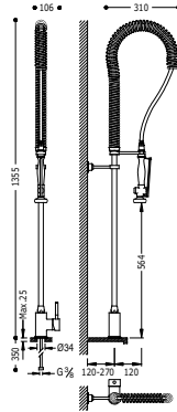
Monomando fregadero vertical
