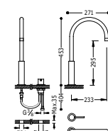
Monomando de repisa STUDY
