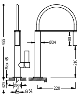
Monomando fregadero vertical CLASS con rociador extraíble
