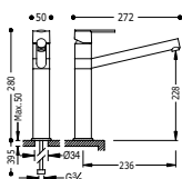
Monomando fregadero vertical LEX caño largo
