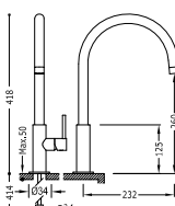
Monomando fregadero vertical MAX
