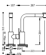
Monomando fregadero vertical LEX con ducha extraíble (2 funciones)
