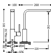
Monomando fregadero vertical CUADRO caño de 35x15 mm.
