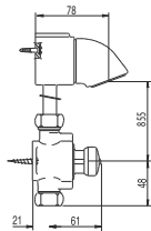
Conjunto de ducha grifo más rociador
