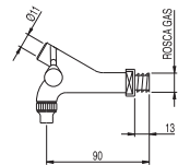
Grifo de vino Nº 1/N
