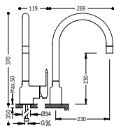
Monomando fregadero vertical con rociador extraíble
