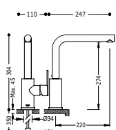
Monomando fregadero vertical LEX-TRES
