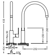
Monomando fregadero vertical LOFT-TRES
