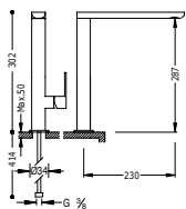
Monomando fregadero vertical LOFT-TRES caño de 34x15 mm.
