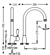
Monomando fregadera vertical RETRO-TRES con rociador extraíble
