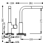
Monomando fregadero vertical CUADRO-TRES con ducha extraíble
