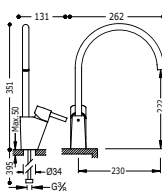
Monomando fregadero vertical ALPLUS
