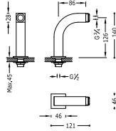
Codo adaptador baño-ducha 2 unidades con silenciador
