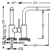
Monomando fregadero vertical MAX-TRES con ducha extraíble
