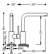
Monomando fregadero vertical MAX
