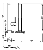
Monomando fregadero vertical MAX-TRES caño de 34x9 mm.
