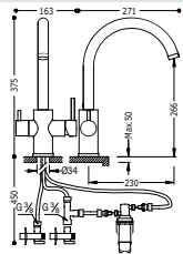
Monomando fregadera vertical ECOSMOSIS doble función con filtro
