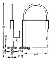
Monomando fregadero vertical CUADRO-TRES con rociador extraíble
