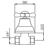
Llave de paso 3/4"
