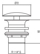
Válvula lavabo libre (desagüe siempre abierto) Tapón Ø 72 mm
