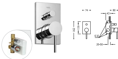
Monomando empotrar (2 vías) cuerpo empotrado incluido
