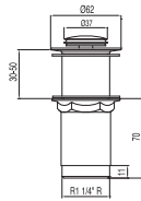
Válvula lavabo sin rebosadero Tapón Ø 37 mm CLICK-CLACK
