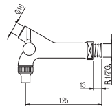
Grifo de vino Nº 2/N
