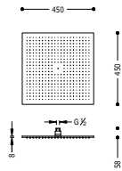
Rociador ducha anticalcárea 450x450 mm.
