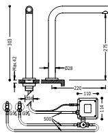
Fregadera electrónica mezclador TOUCH-TRES Sistema sensible al tacto. Sólo tocar (NO pulsar). NOTA: Incluye un grifo mezclador dos aguas con tubos flexibles (ref. 1.92.507.30).
