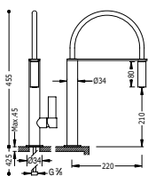
Monomando fregadero vertical CLASS-TRES con rociador extraíble
