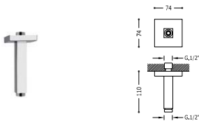
Brazo techo para rociador ducha
