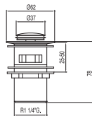
Válvula lavabo con rebosadero Tapón Ø 37 mm CLICK-CLACK
