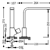
Monomando fregadero vertical CUADRO caño de 35x15 mm.
