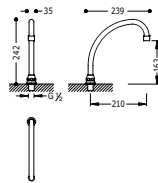
Caño fregadero con enlace
