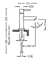
Monomando lavabo Ø 30 mm.
