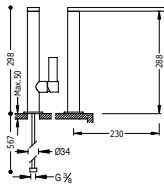
Monomando fregadero vertical CLASS caño de 34x9 mm.
