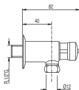
Grifo de urinario
