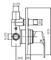
Monomando empotrar (2 vías) cuerpo empotrado incluido
