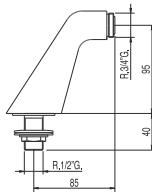
Codo adaptador baño-ducha 2 unidades con silenciador
