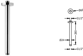
Brazo techo para rociador ducha
