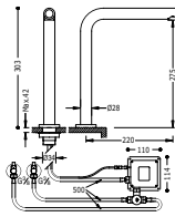
Lavabo electrónico mezclador TOUCH-TRES Sistema sensible al tacto. Sólo tocar (NO pulsar). NOTA: Incluye un grifo mezclador dos aguas con tubos flexibles (ref: 1.92.507.30).
