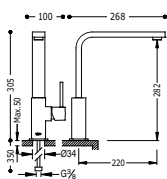
Monomando fregadero vertical CUADRO-TRES caño de 35x15 mm.
