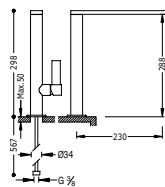
Monomando fregadero vertical CLASS-TRES caño de 34x9 mm.
