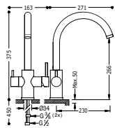
Monomando fregadera vertical ECOSMOSIS doble función sin filtro. NOTA: para instalaciones de osmosis.
