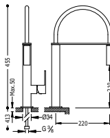
Monomando fregadero vertical CUADRO con rociador extraíble.
