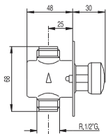
Grifo de urinario para empotrar
