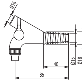
Grifo de vino Nº 1/C
