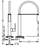
Monomando fregadero vertical MAX-TRES con rociador extraíble
