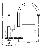
Monomando fregadero vertical LOFT
