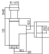
Sifón lavabo visto cuadrado telescópico
