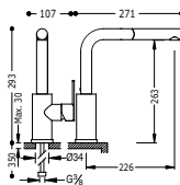
Monomando fregadero vertical LEX-TRES con ducha extraíble
