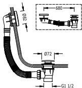
Desagüe bañera con rebosadero Tapón Ø 72 mm CLICK-CLACK
