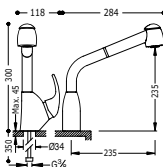
Monomando fregadero vertical con ducha extraíble (2 funciones)
