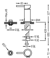
Monomando bidé con duchita
