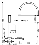
Monomando fregadero vertical CLASS con rociador extraíble.
