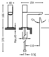
Grifo lavabo 1 agua o premezclada
