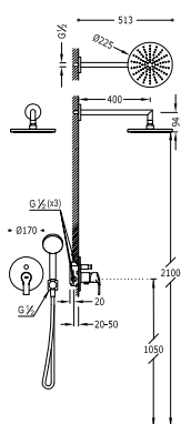
Kit de ducha monomando empotrado con cierre y regulación de caudal. · Cuerpo empotrado incluido · Ducha fija Ø 225 mm. con rótula. (299.632.01). · Soporte con toma pared (205.182.01). · Ducha móvil masaje Ø 110 mm. (5 funciones). · Flexo SATIN (91.34.609.15).
