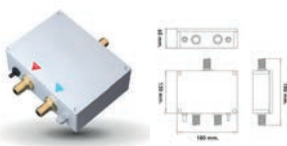
Mezclador transformador ref.9905000 Transformer mixer
